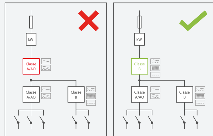
Instalação correcta dos equipamentos de protecção de Classe B.
