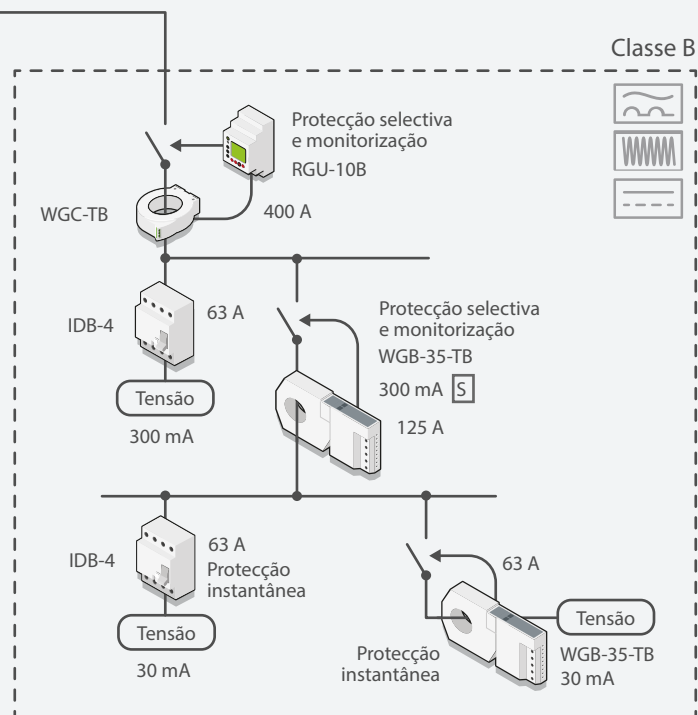
Instalação correcta dos equipamentos de protecção de Classe B.
